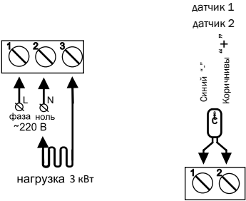
Схема подключения
