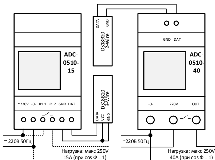
Рис. 1. Схема подключения
